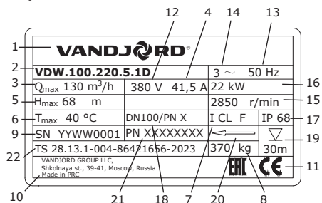
Рис. 5 Фирменная табличка
