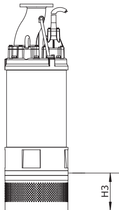
Рис. 12 Минимальный уровень воды
