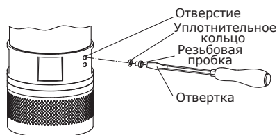
Рис. 14 Отверстие для слива и заливки масла
