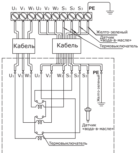
Рис. 11 Схема подключения «звезда-треугольник» для насосов VDW мощностью 90, 110 кВт
