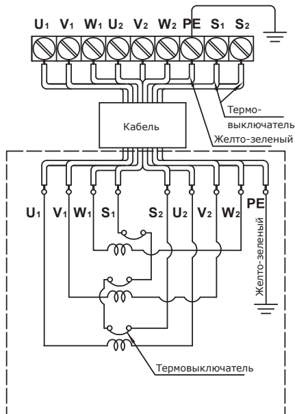
Рис. 9 Схема подключения «звезда-треугольник» для насосов VDW мощностью 22–45 кВт
