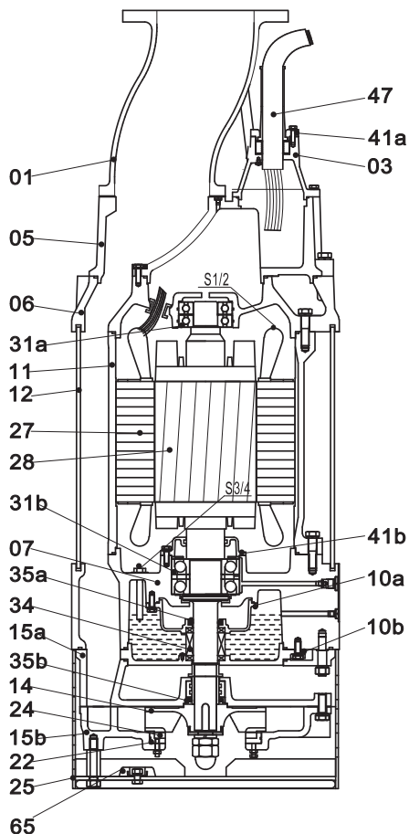
Рис. 3 Продольный разрез насоса VDW, 55–110 кВт (кроме высоконапорного VDW.150.1100.5.1D)
