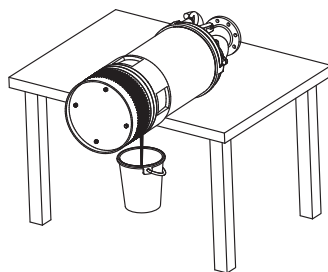
Рис. 15 Слив масла
