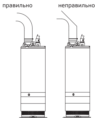
Рис. 7 Правильность подсоединения шланга
