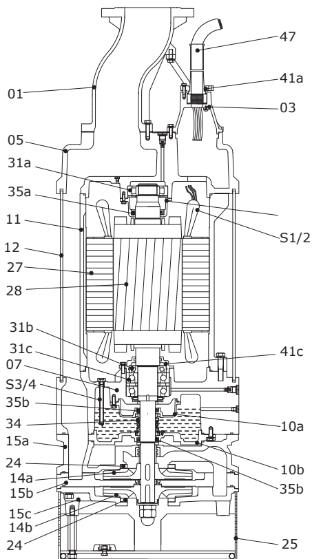
Рис. 4 Продольный разрез насоса VDW, высоконапорные VDW.100.370.5.1D, VDW.150.1100.5.1D
