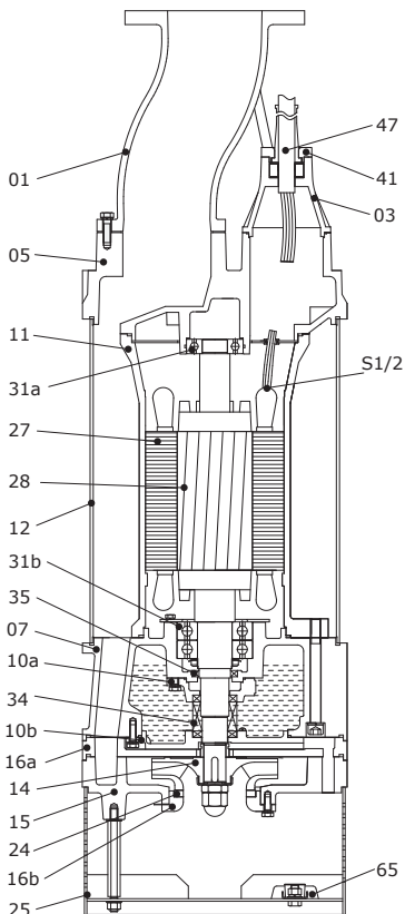
Рис. 1 Продольный разрез насоса VDW, 22–30 кВт
