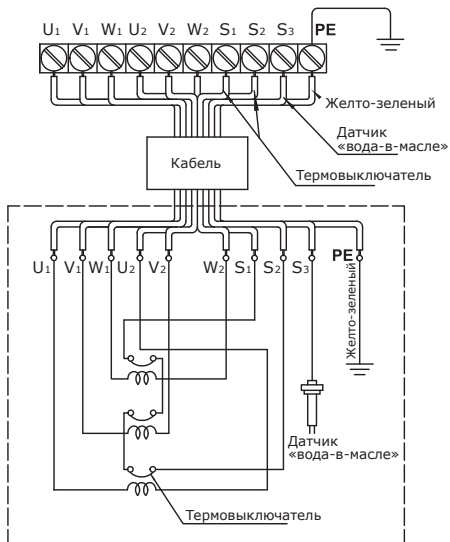
Рис. 10 Схема подключения «звезда-треугольник» для насосов VDW мощностью 55, 75 кВт
