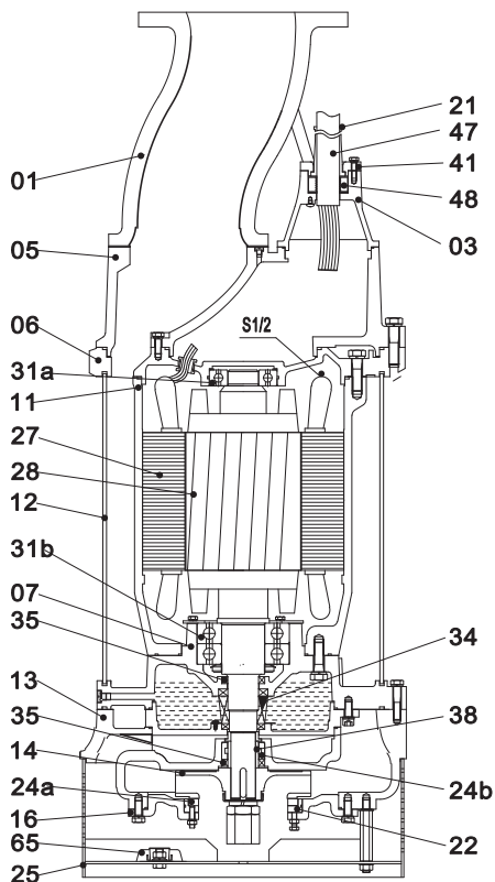
Рис. 2 Продольный разрез насоса VDW, 37–45 кВт (кроме высоконапорного VDW.100.370.5.1D)
