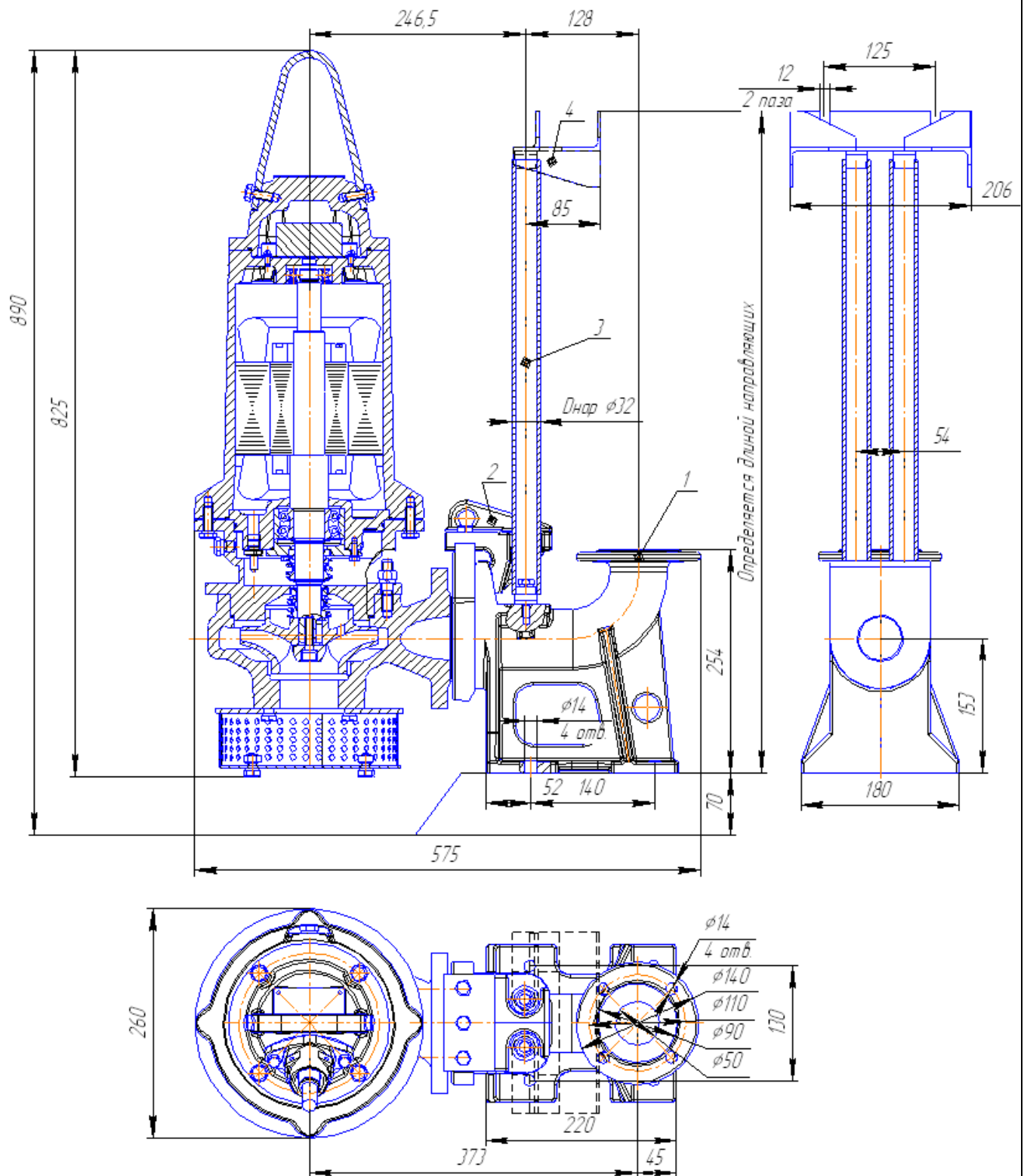
Рис. 38 Общий вид и габаритные размеры электронасоса "Иртыш"
