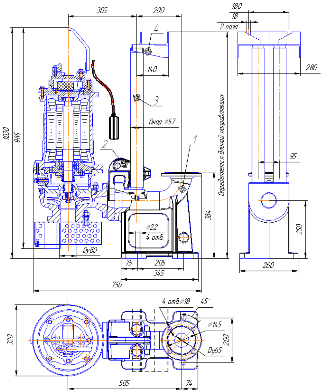
Рис. 36 Общий вид и габаритные размеры электронасоса "Иртыш"
