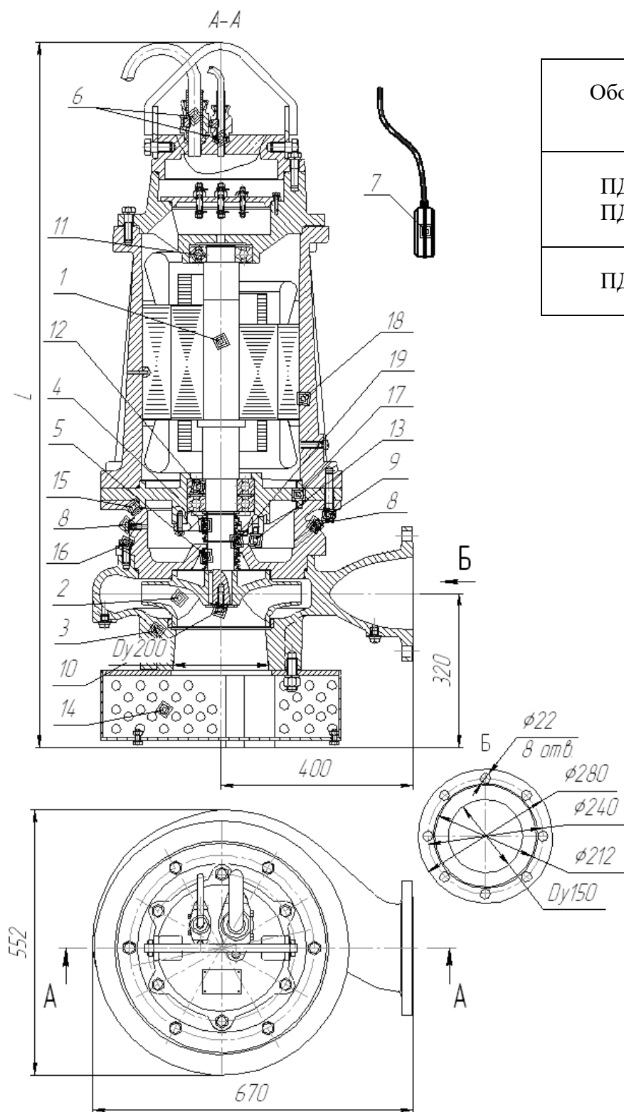
Рис. 32 Общий вид, габаритные и присоединительные размеры электронасоса "Иртыш" ПД 150/315 – 37/4; ПД 150/315 – 45/4; ПД 150/315 – 55/4.
