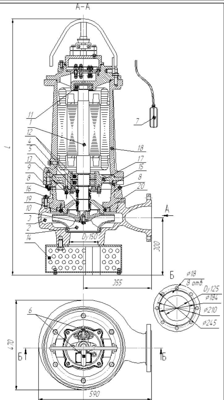
Рис. 29 Общий вид, габаритные и присоединительные размеры электронасоса "Иртыш" ПД 125/315 – 18,5/4 ПД 125/315 – 30/4
