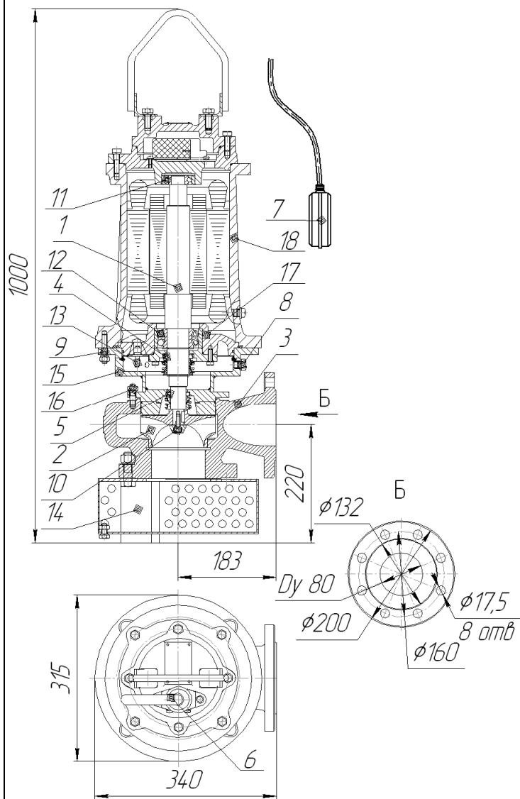
Рис. 24 Общий вид, габаритные и присоединительные размеры электронасоса "Иртыш" ПД 80/125 – 11/2
