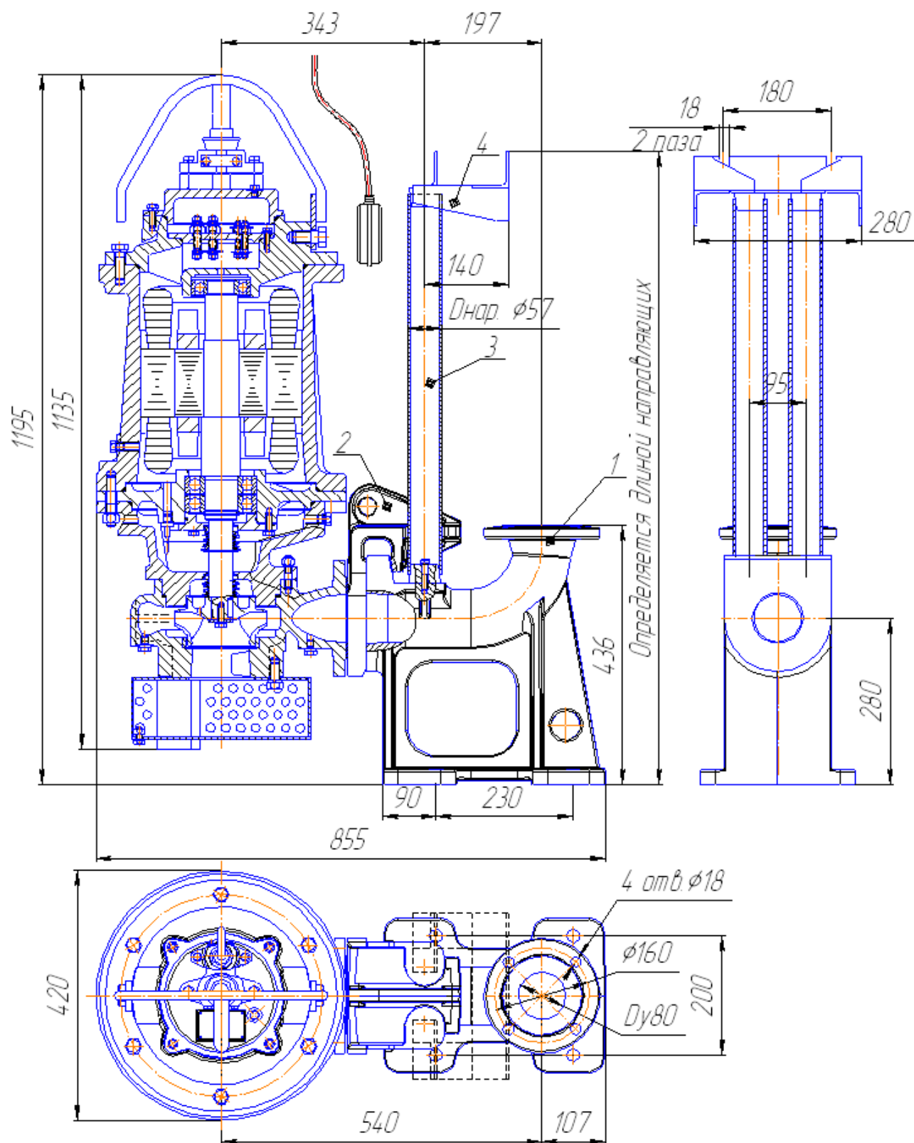
Рис. 46 Общий вид и габаритные размеры электронасоса "Иртыш" ПД 80/160 – 15/2 с опускающим устройством. 1. Патрубок погружной; 2. Насос с захватом; 3. Направляющие; 4. Кронштейн.
