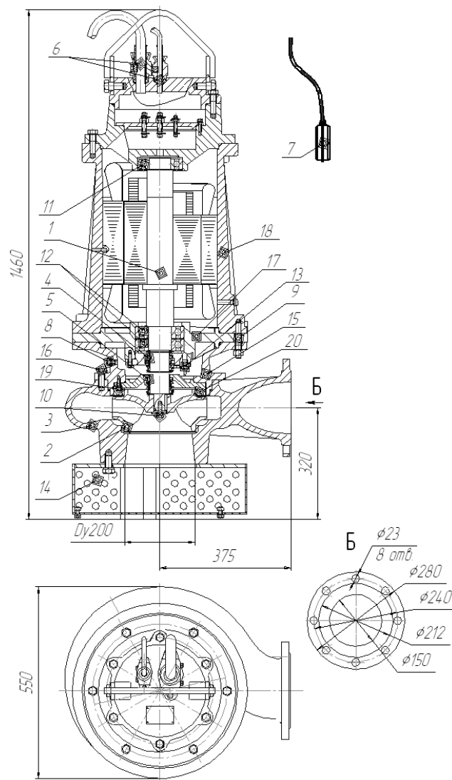
Рис. 31 Общий вид, габаритные и присоединительные размеры электронасоса "Иртыш" ПД 150/250 – 37/4
