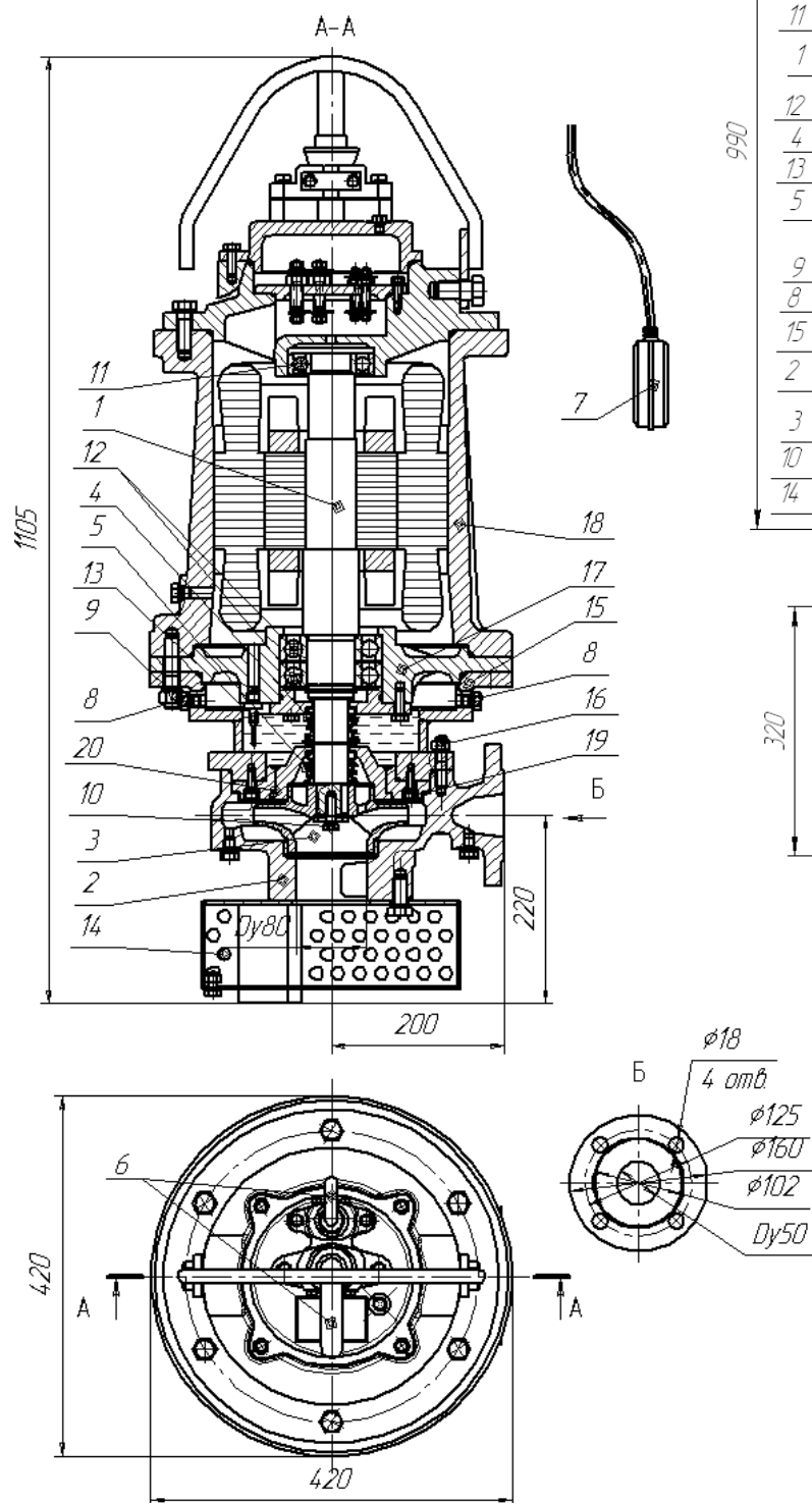
Рис. 19 Общий вид, габаритные и присоединительные размеры электронасоса "Иртыш" ПД 50/200 – 15/2
