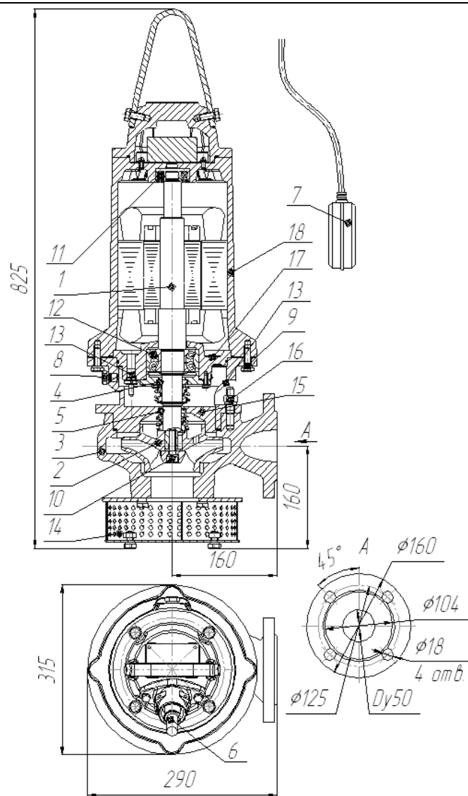
Рис. 18 Общий вид, габаритные и присоединительные размеры электронасоса "Иртыш" ПД 50/160 – 4/2
