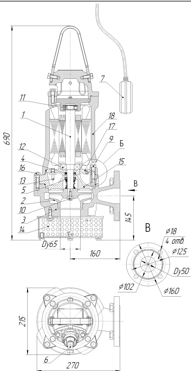
Рис. 17 Общий вид, габаритные и присоединительные размеры электронасоса "Иртыш" ПД 50/125 – 3/2
