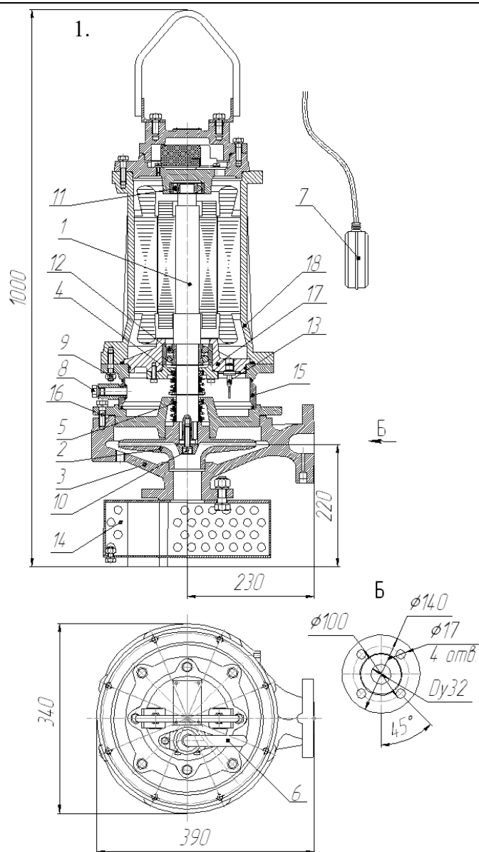
Рис. 15 Общий вид, габаритные и присоединительные размеры электронасоса "Иртыш" ПД 32/250 – 11/2
