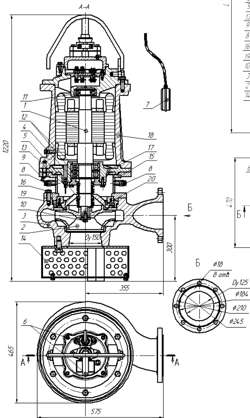
Рис. 28 Общий вид, габаритные и присоединительные размеры электронасоса "Иртыш" ПД 125/250 – 15/4
