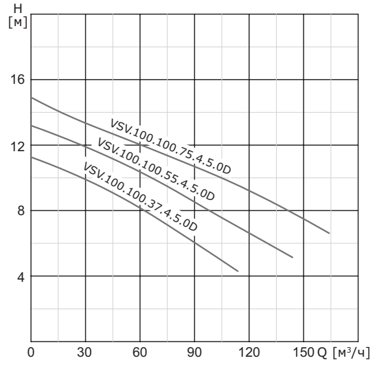
VSV.100 (4-полюсные)
