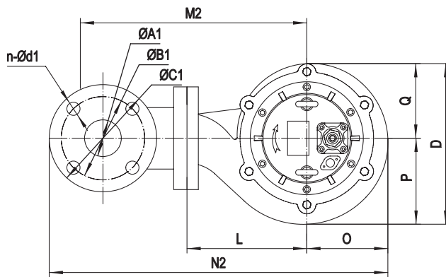
Фланцевое соединение с коленом
