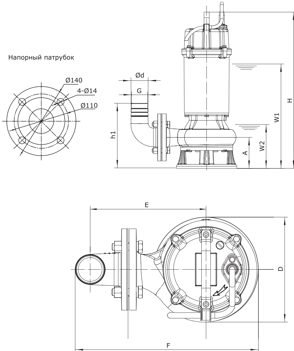
Рис. 19 Габаритные размеры насосов VSL.50.075.2.5.0D.T и VSL.50.15.2.5.0D.T
