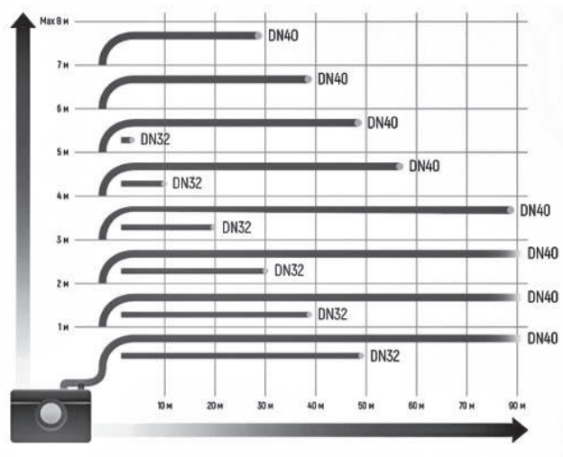
Рис. 33 Максимальная длина напорного трубопровода
