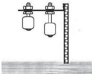
Рис. 29 Монтаж поплавкового выключателя MS K1
